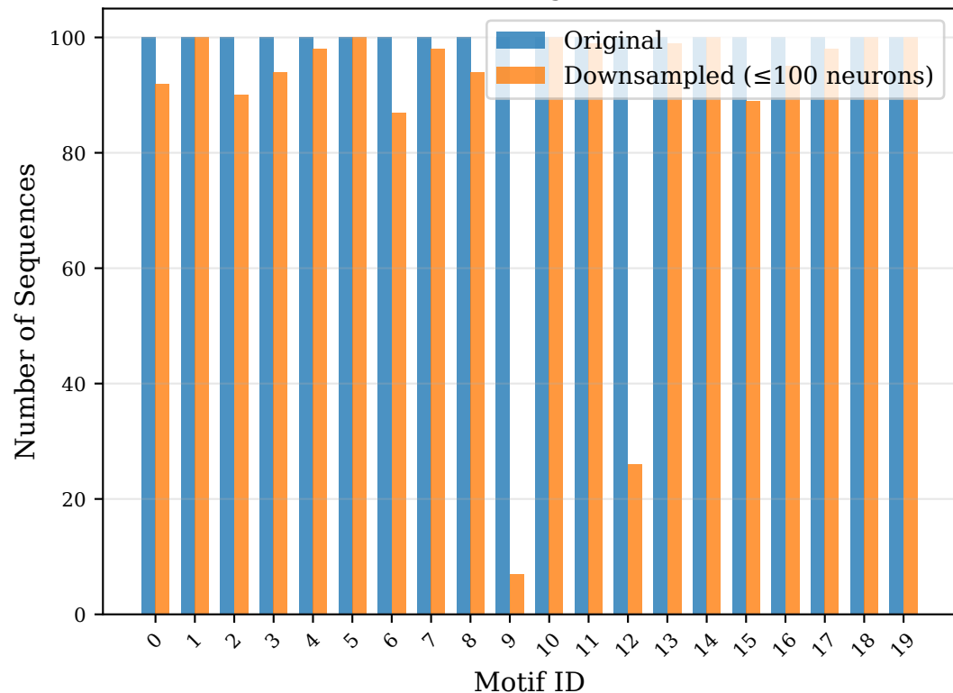
Neuron Participation - Original
